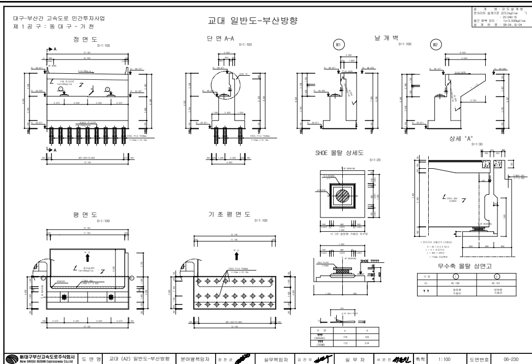
<교대 일반도>
