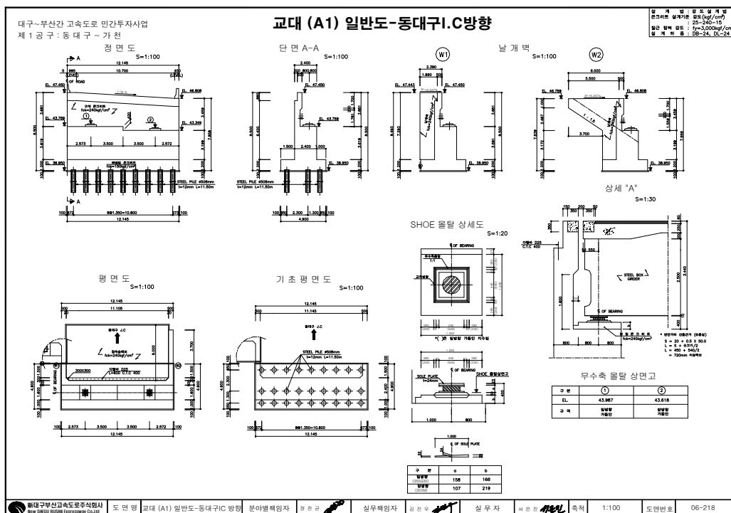
〈교대 일반도〉
