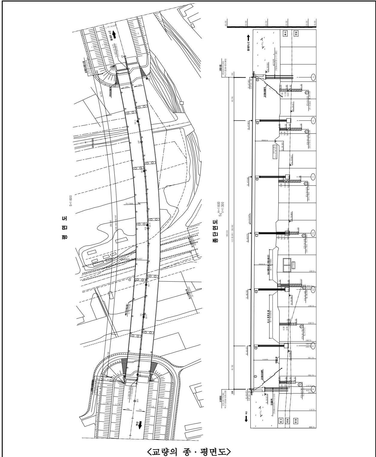
【그림 1.4.1】 용계2교(대구) 종·평면도
