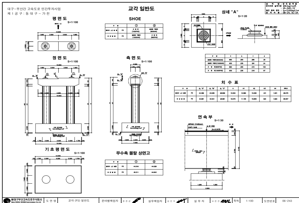
<교각 일반도>
