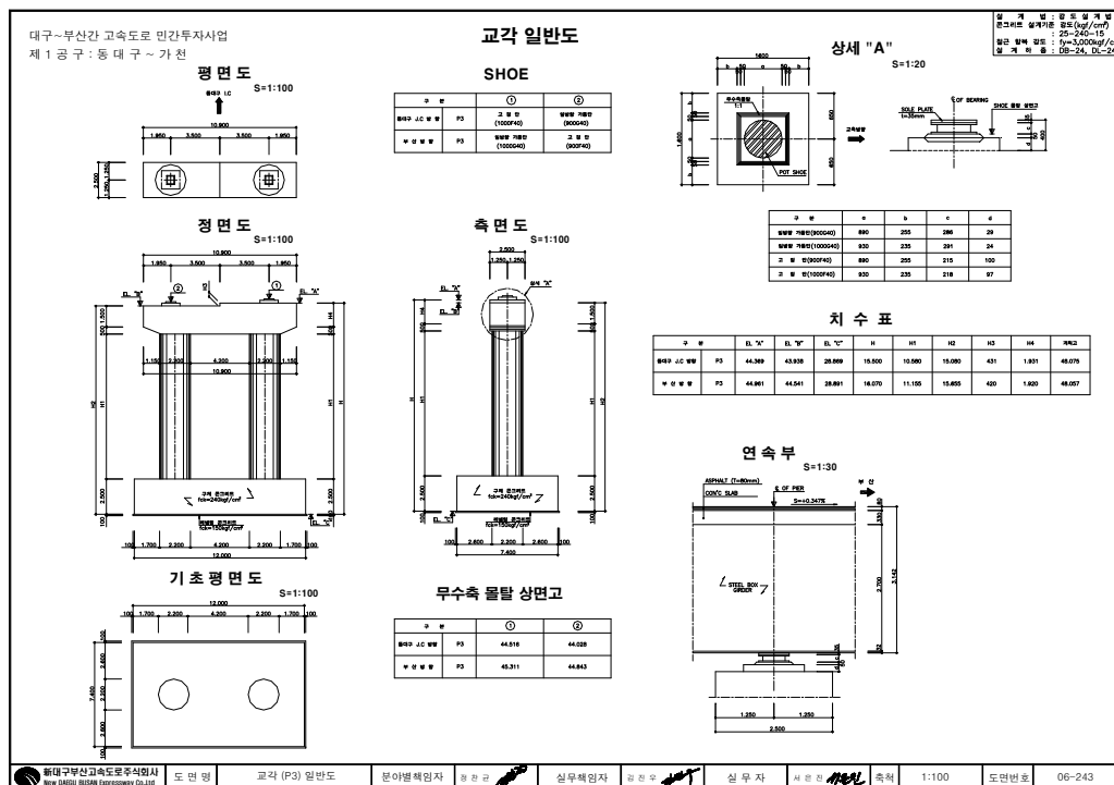
〈교각 일반도〉
