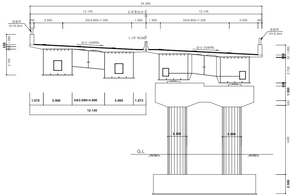
<교량 횡단면도>
